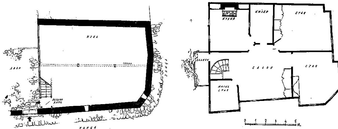
Фиг. 67. Къща на Васил Ламбринов. План приземие и жилищен етаж по арх. Иванчев (Иванчев, 1957)
