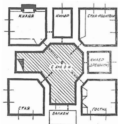
Фиг. 59. План на етажа на напълно развитата несебърска възрожденска къща (Иванчев, 1957)
