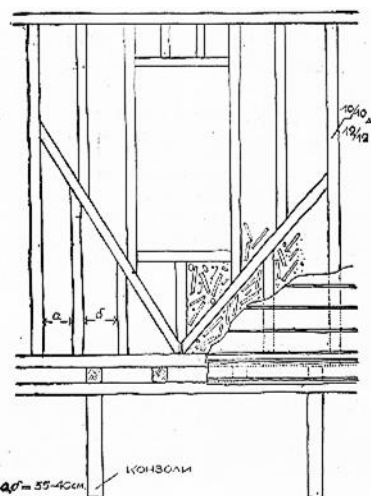
Фиг. 83. Разположение на прозорец в скелета на паянтова конструкция (Иванчев, 1957)
