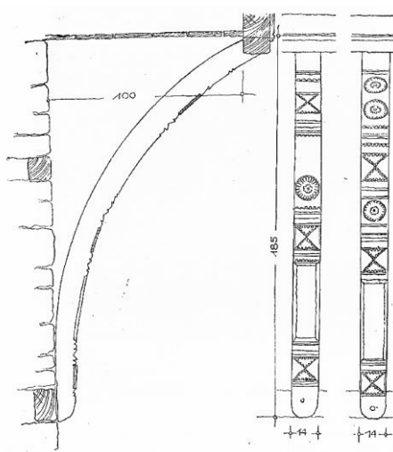
Фиг. 88. Дървен подкос на къщата на В. Ламбринов (диахронен анализ 1957 и 2023). Чертеж на дървен подкос (Иванчев, 1957)
