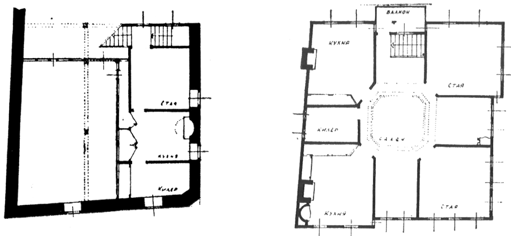
Фиг. 73. Къща на Аргир Пиков и Катина Янулова. План приземие и жилищен етаж по арх. Иванчев (Иванчев, 1957)
