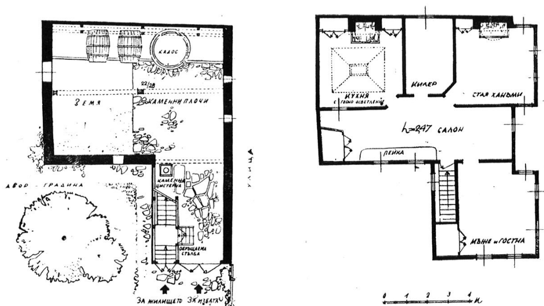
Фиг. 69. Къща на Зоица Янулова. План приземие и жилищен етаж по арх. Иванчев (Иванчев, 1957)
