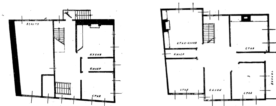
Фиг. 71. Къща на Димитър Русиев и Олга Грамадска. План приземие и жилищен етаж по арх. Иванчев (Иванчев, 1957)
