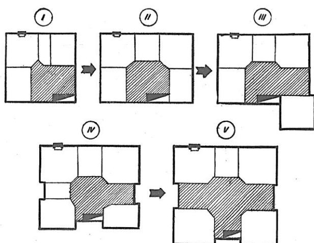
Фиг. 58. Схема на развитието на Черноморската къща на арх. Иванчев (Иванчев, 1957)
