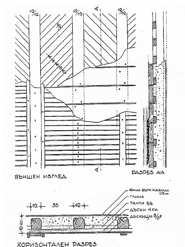
Фиг. 84. Конструкция на паянтова стена в стара несебърска къща (Иванчев, 1957)
