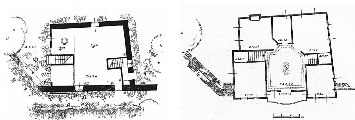
Фиг. 65. Къща на Желю Богданов. План приземие и жилищен етаж по арх. Иванчев (Иванчев, 1957)
