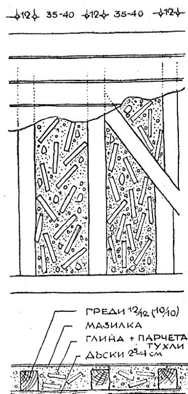
Фиг. 85. Конструкция на паянтова стена в нова несебърска къща (Иванчев, 1957)
